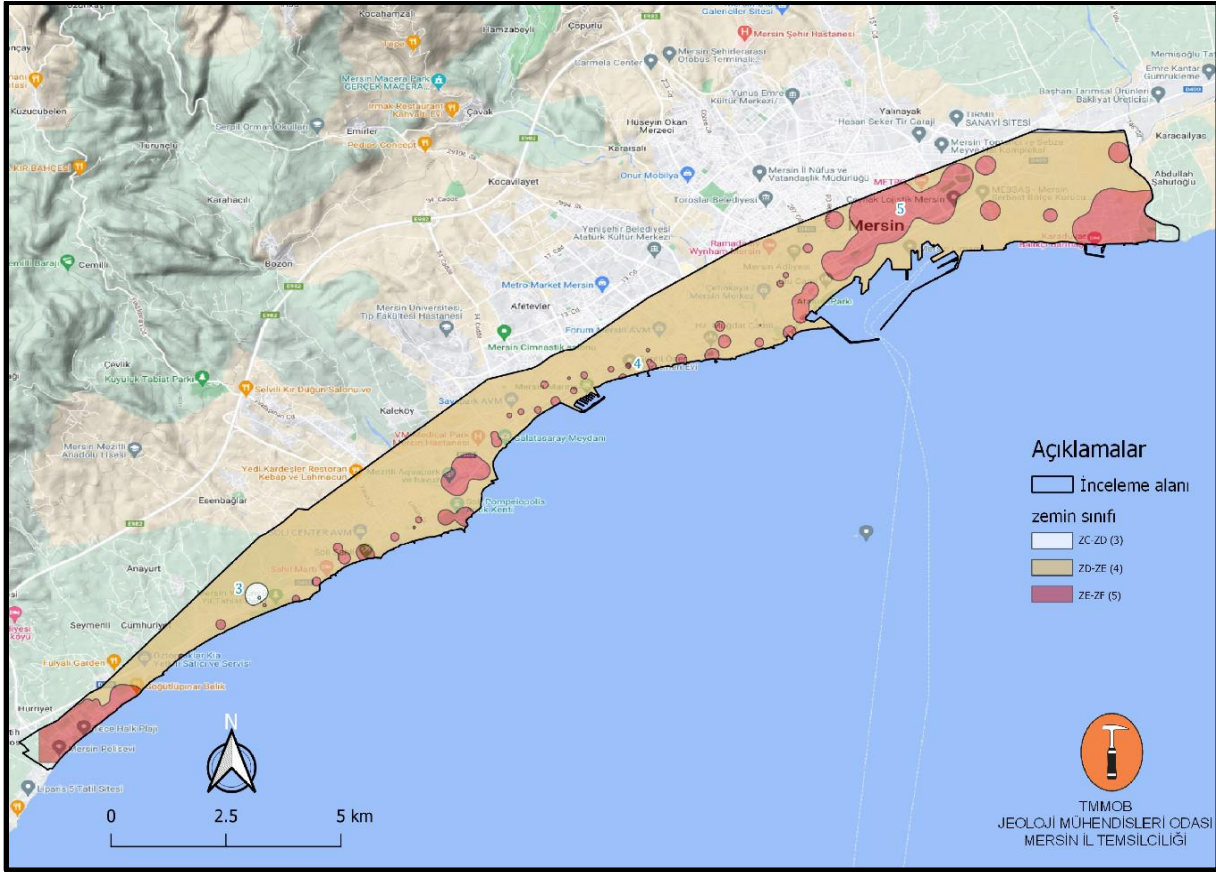
Şekil 6. İnceleme alanı zeminlerinin TBKY 2018 baz alınarak ağırlıklandırılmış zemin sınıfı dağılım haritası.
