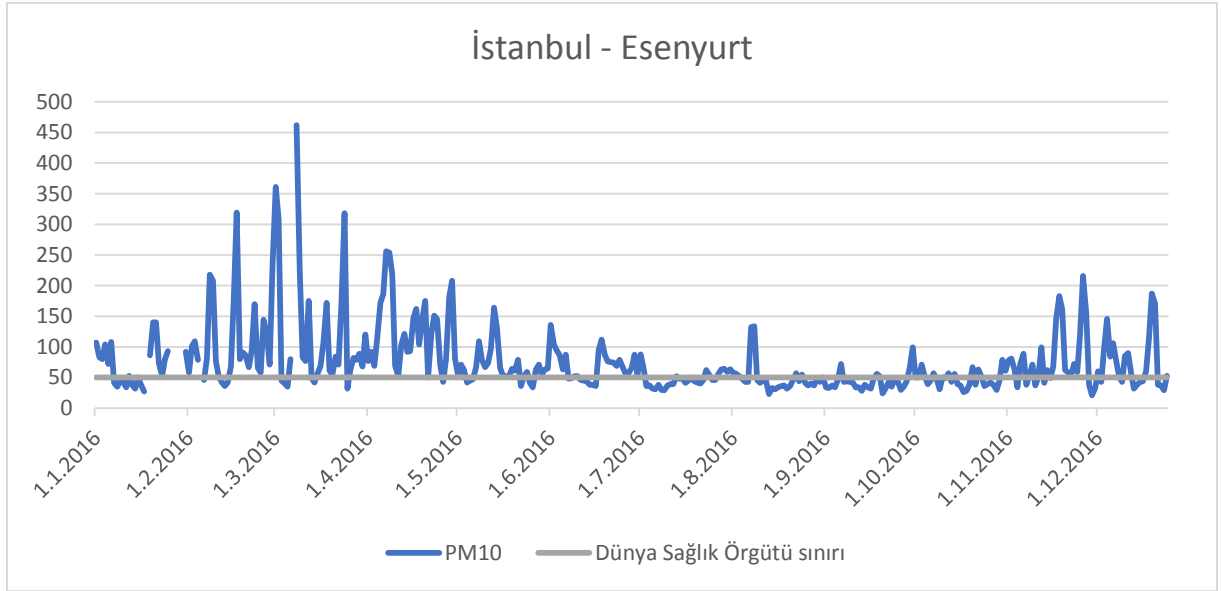
Şekil 8: WHO-DSÖ sınır değeri ve ölçüm sonuçlarının yıl içinde dağılımı (İstanbul-Esenyurt). (T.C. Çevre ve Şehircilik Bakanlığı, 2016)
