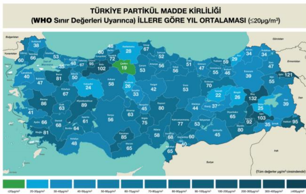
Şekil 1: PM10 Ölçümlerinin Yıllık Ortalaması: ( 20 \mu\text{g}/\text{m}^3 )
