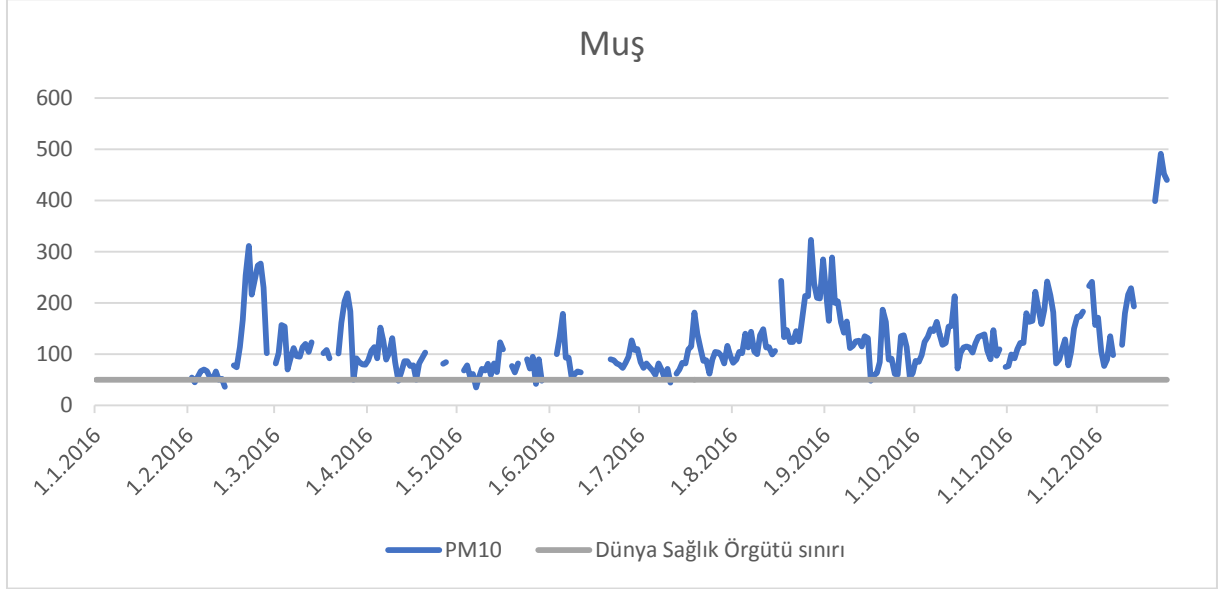
Şekil 14: WHO-DSÖ sınır değeri ve ölçüm sonuçlarının yıl içinde dağılımı (Muş). (T.C. Çevre ve Şehircilik Bakanlığı, 2016)
