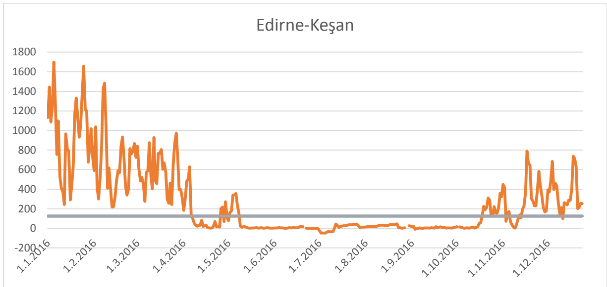
Şekil 6: WHO-DSÖ sınır değeri ve ölçüm sonuçlarının yıl içinde dağılımı” SO2” (Edirne-Keşan) (T.C. Çevre ve Şehircilik Bakanlığı, 2016)
