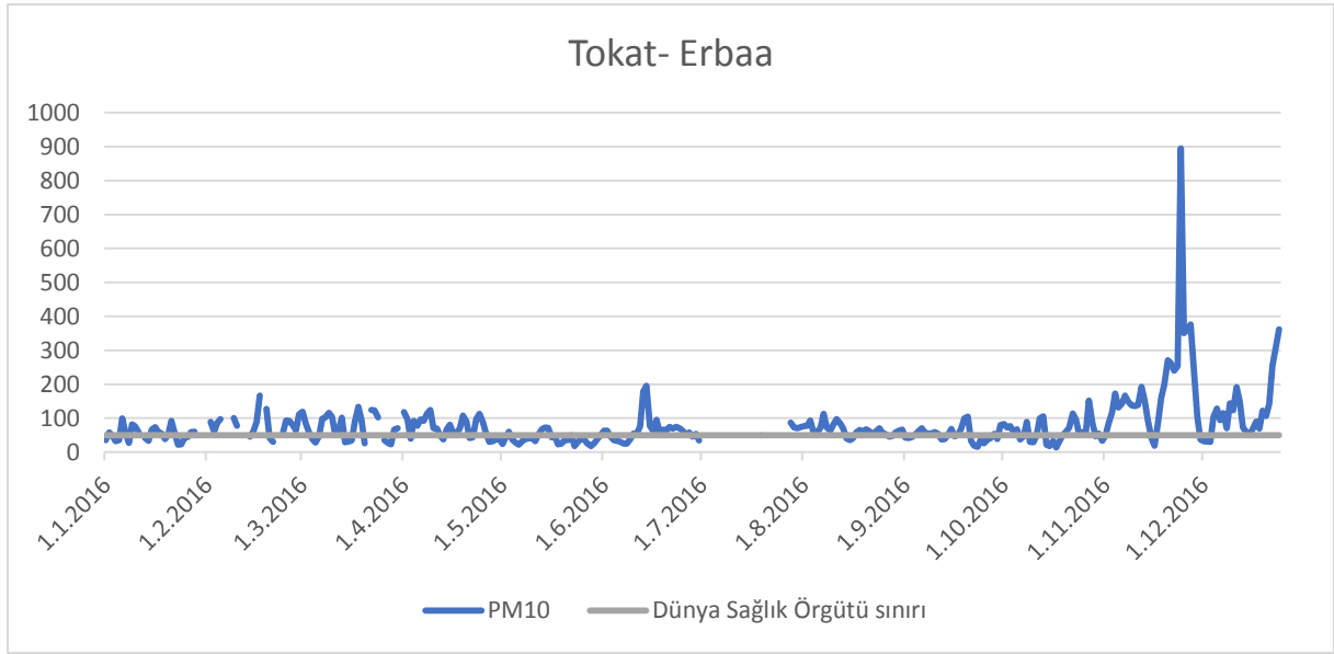
Şekil 15: WHO-DSÖ sınır değeri ve ölçüm sonuçlarının yıl içinde dağılımı (Tokat-Erbağ). (T.C. Çevre ve Şehircilik Bakanlığı, 2016)
