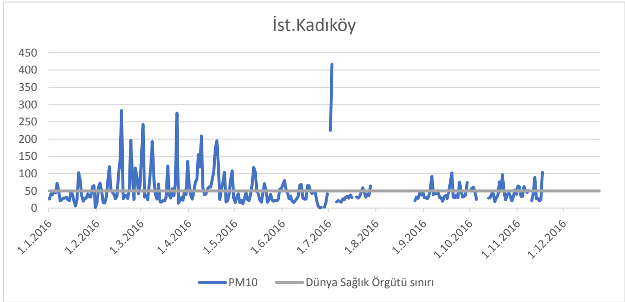
Şekil 9: WHO-DSÖ sınır değeri ve ölçüm sonuçlarının yıl içinde dağılımı (İstanbul-Kadıköy) (T.C. Çevre ve Şehircilik Bakanlığı, 2016)
