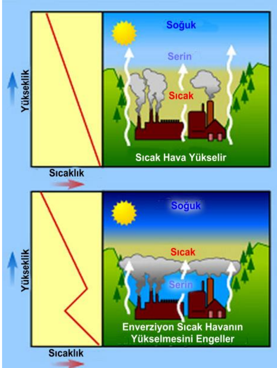
Şekil 2: Enverziyon (T.C. ORMAN VE SU İŞLERİ BAKANLIĞI Meteoroloji Genel Müdürlüğü, 2016)
