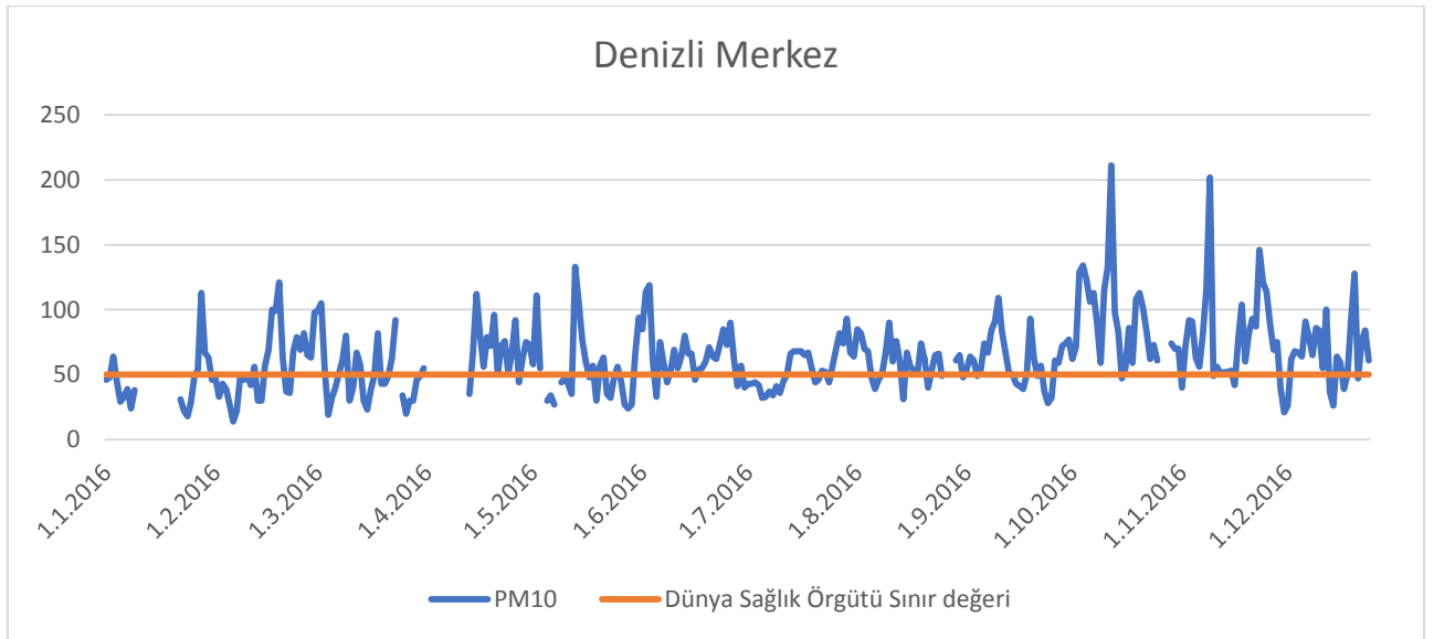
Şekil 16: WHO-DSÖ sınır değeri ve ölçüm sonuçlarının yıl içinde dağılımı (Denizli-Merkez). (T.C. Çevre ve Şehircilik Bakanlığı, 2016)
