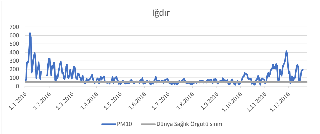
Şekil 12: WHO-DSÖ sınır değeri ve ölçüm sonuçlarının yıl içinde dağılımı (İğdır ili). (T.C. Çevre ve Şehircilik Bakanlığı, 2016)
